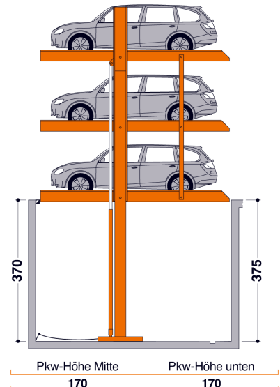
MultiBase G63-370 (Aufstellung im Freien)
