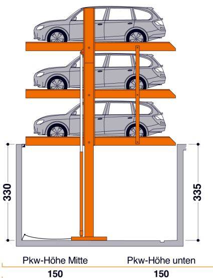
MultiBase G63-330 (Aufstellung im Freien)
