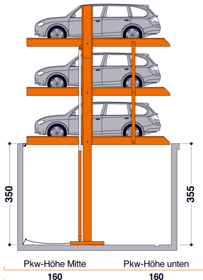
MultiBase G63-350 (Aufstellung im Freien)
